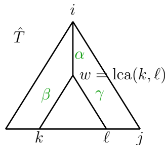
Abbildung 2.38: Skizze: Abstände im gewurzelten additiven Baum \hat{T}
