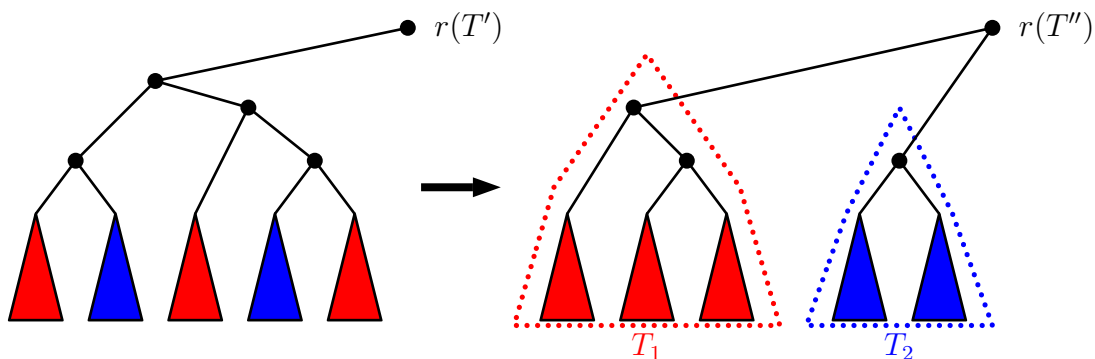
Abbildung 2.72: Skizze: Umbau des niedrigen ultrametrischen Baumes
