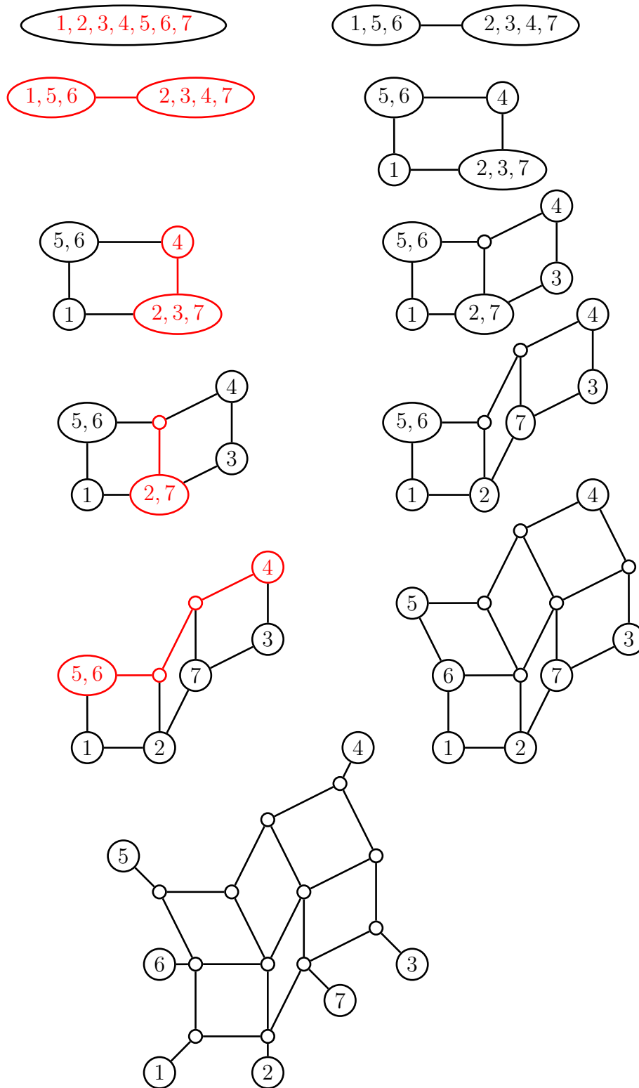
Abbildung 2.102: Beispiel: Konstruktion eines Split Graphen
