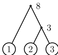
Abbildung 2.40: Gegenbeispiel: D nicht additiv, aber D' ultrametrisch
