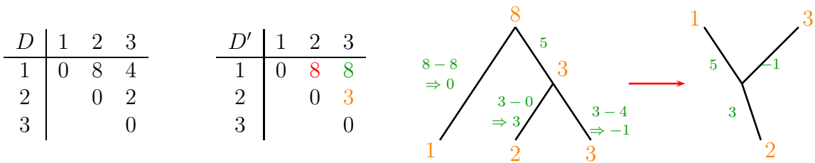
Abbildung 2.43: Gegenbeispiel: D nicht additiv und D' ultrametrisch (Fortsetzung)
