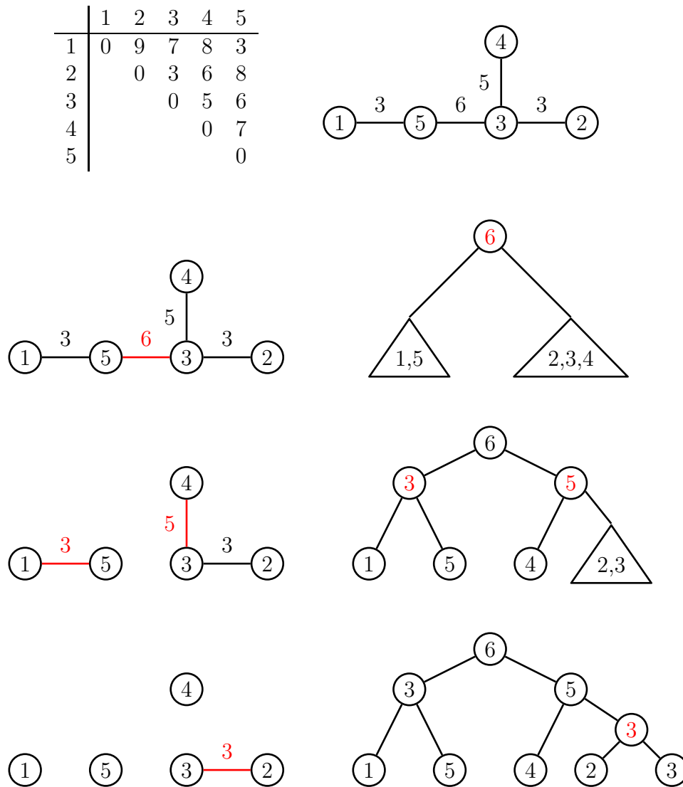
Abbildung 2.68: Beispiel: Konstruktion eines höchsten ultrametrischen Baumes
