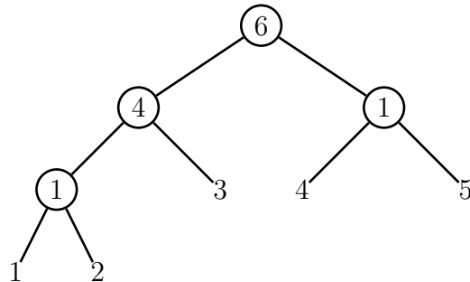
Abbildung 2.74: Beispiel: Einfache Lösung des ultrametrischen Sandwich-Problems
