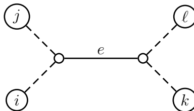
Abbildung 2.97: Skizze: Kante e im additiven Baum T(D)
