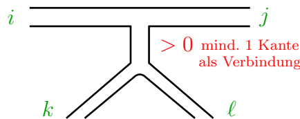
Abbildung 2.46: Skizze: Die Pfade i \rightarrow j und k \rightarrow \ell sind knotendisjunkt
