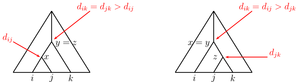
Abbildung 2.23: Skizze: Fall 1 und Fall 2
