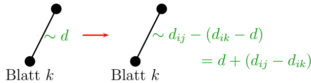
Abbildung 2.37: Skizze: Verlängern der zu Blättern inzidenten Kanten
