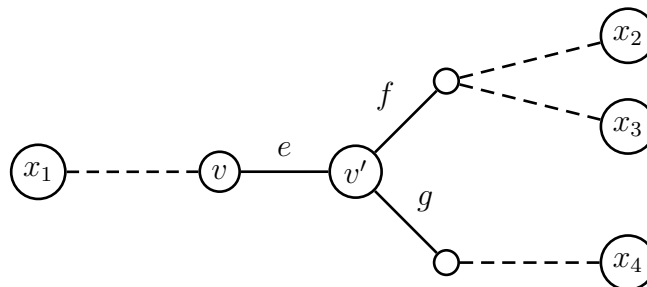
Abbildung 2.86: Skizze: Annahme S \neq \Sigma(f)
