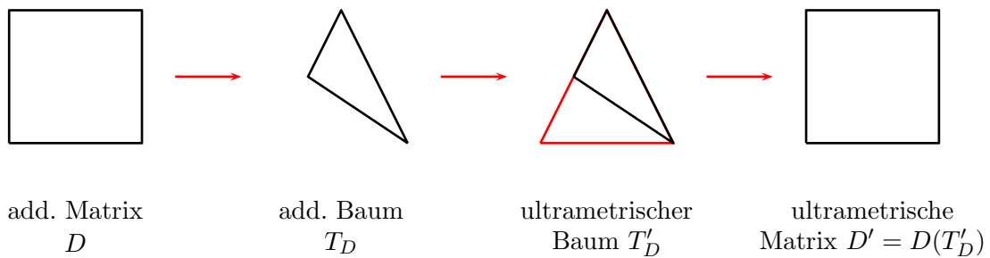
Abbildung 2.35: Skizze: Schema der Transformation einer additiven Matrix in eine ultrametrische Matrix
