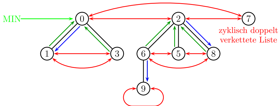
Abbildung 2.54: Beispiel: Fibonacci-Heap
