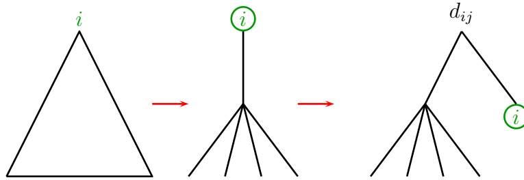
Abbildung 2.39: Skizze: Wirkliches Wurzeln des additiven Baumes
