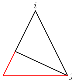
Abbildung 2.36: Skizze: Wurzeln von T_D am Blatt i
