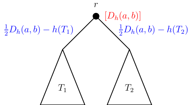
Abbildung 2.66: Skizze: Rekursive Konstruktion eines ultrametrischen Baumes mit Hilfe eines minimalen Spannbaumes
