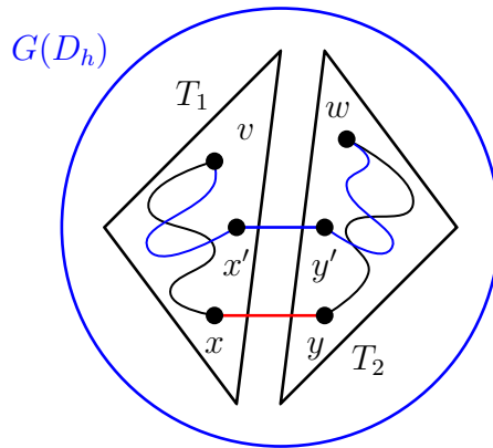
Abbildung 2.75: Skizze: Spannender Wald \{T_1, T_2\} von G(D_h) nach Entfernen von \{x, y\} aus dem minimalen Spannbaum T
