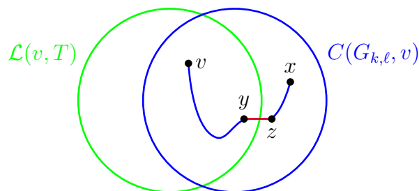
Abbildung 2.71: Skizze: \mathcal{L}(T, v) und C(G_{k,\ell}, v)
