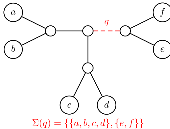
Abbildung 2.82: Beispiel: Ein Split, der durch die Kante q induziert ist
