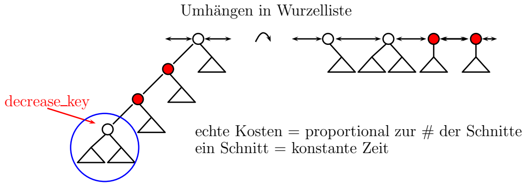
Abbildung 2.61: Skizze: Kosten für decrease_key
